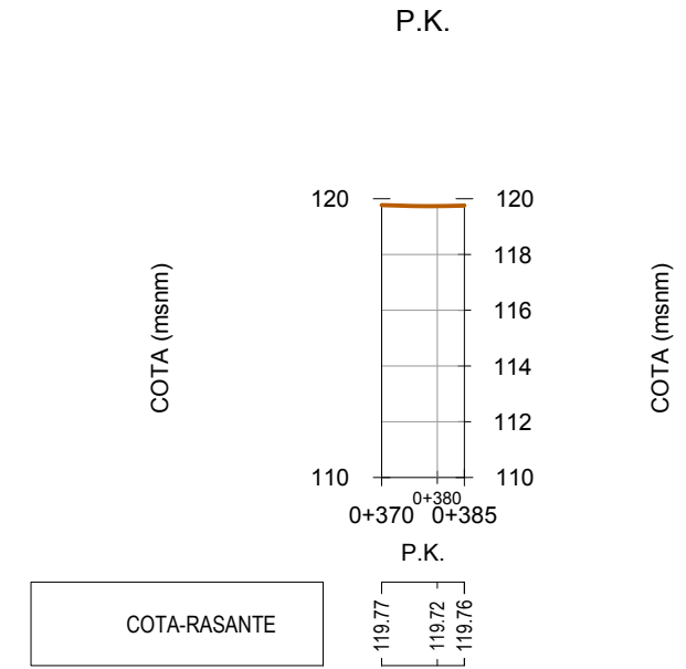
Perfil Longitudinal: Perfil C-6 tramo 2 Escala - V: 200 H:1000
