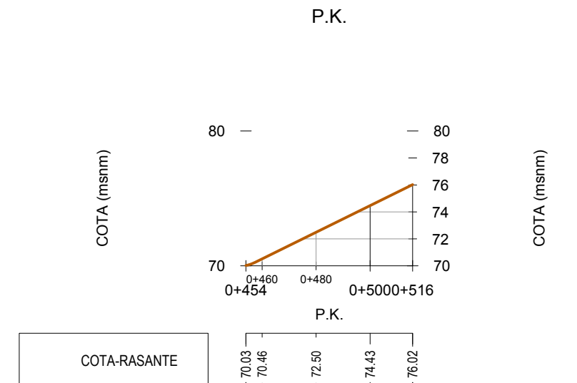
Perfil Longitudinal: Perfil C-3 tramo 3 Escalas - V: 200 H:1000
