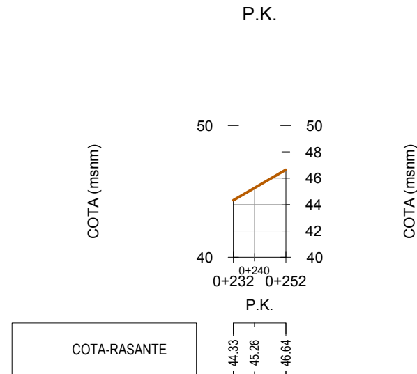
Perfil Longitudinal: Perfil C-3 Tramo 2 Escalas - V: 200 H:1000
