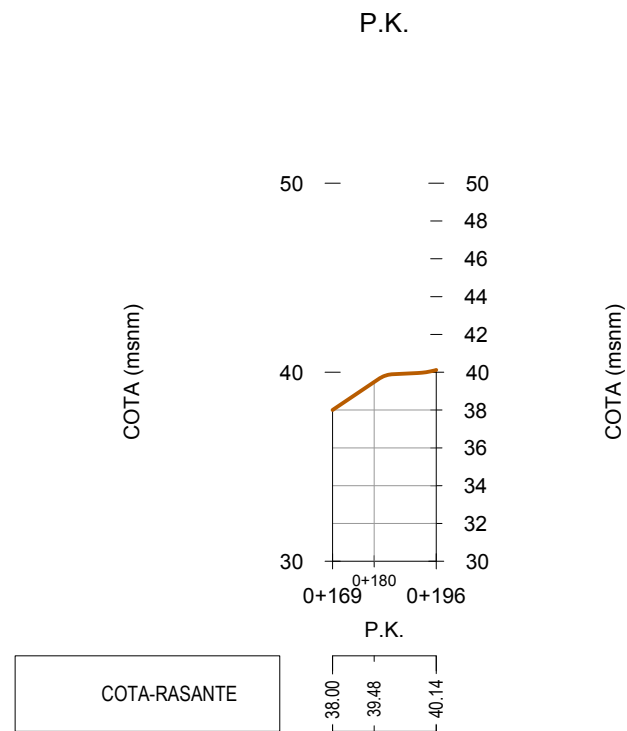
Perfil Longitudinal: Perfil C-3 tramo 1 Escalas - V: 200 H:1000
